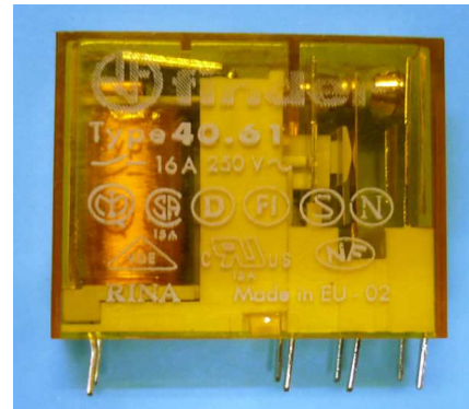
RELÉ AMARILLO
