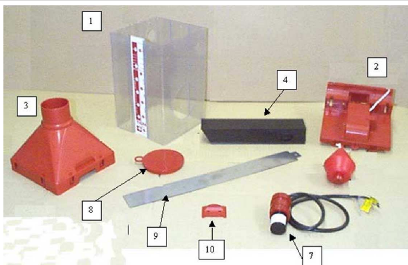
DOSIFICADOR 6 LT.
