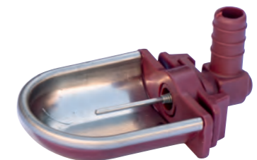
Cod. 10372 Bebedero con válvula acodada
