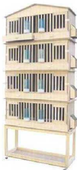
REF.: 072.025 PIE // TERREROS DOBLES-P MEDIDAS: 37 x 77 x 26
